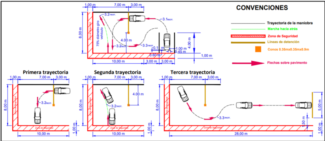
Ilustración 12. Maniobra de cambio de sentido de la marcha en espacio limitado para categorías B1 y C1
